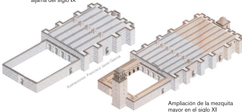
Alzado de la mezquita aljama del siglo IX
